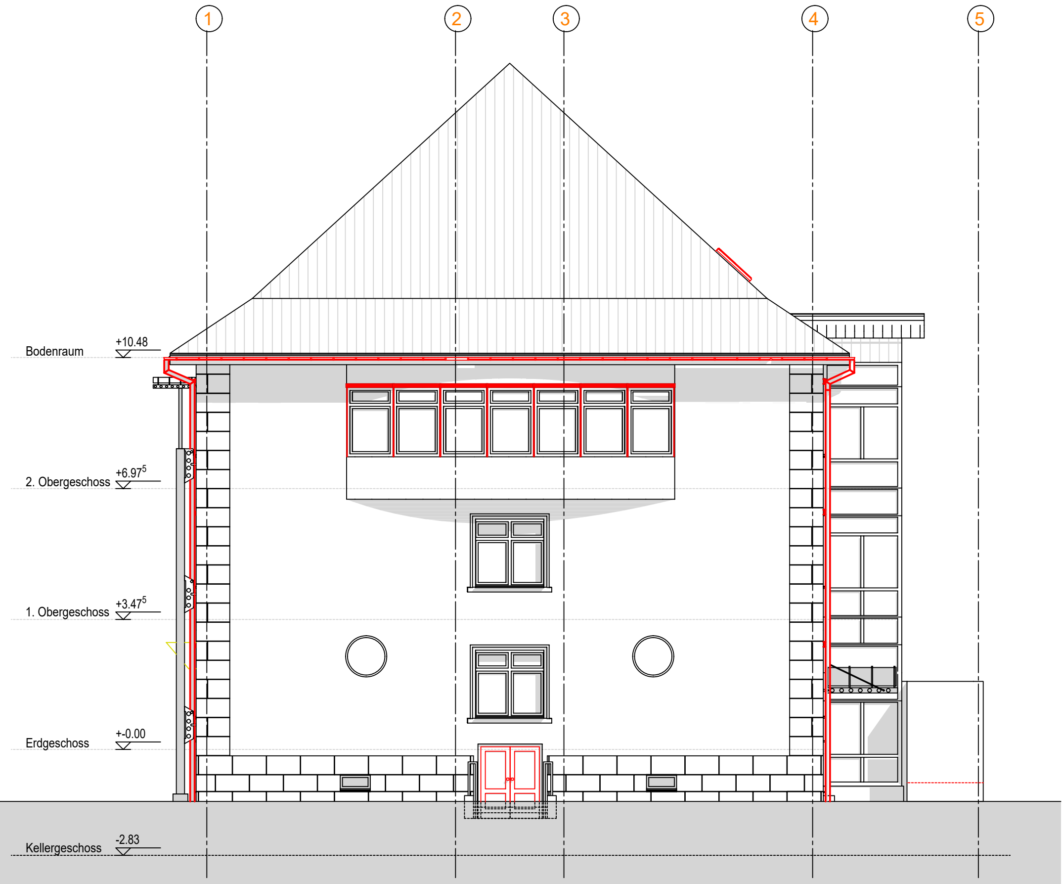
Nordansicht
