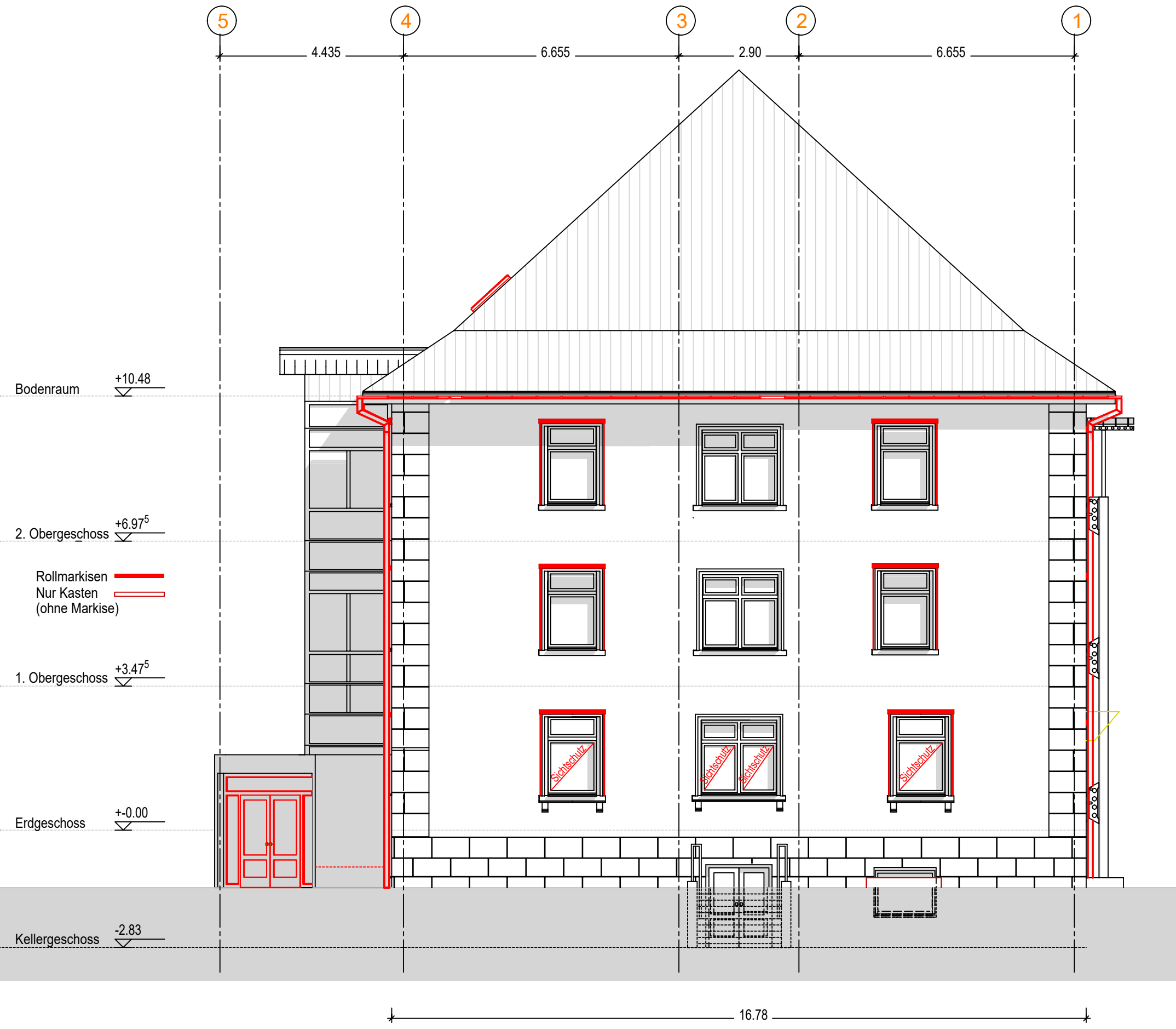
Westansicht
